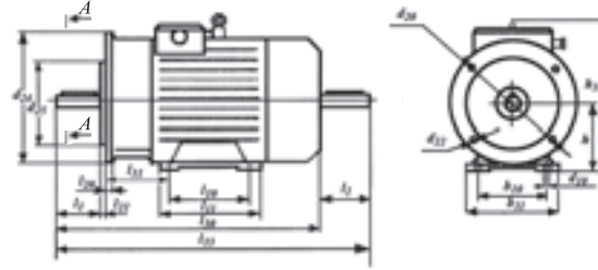
Габаритные, установочные и присоединительные размеры крановых электродвигателей с фазным ротором
